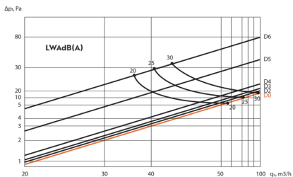
LINEO 500, 20 mm plyšys (oro tiekimas)
