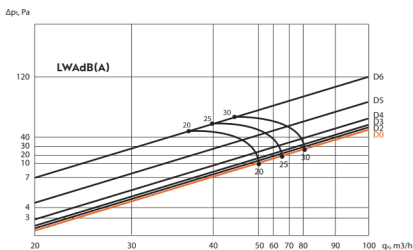
LINEO 500, 20 mm plyšys (oro ištraukimas)
