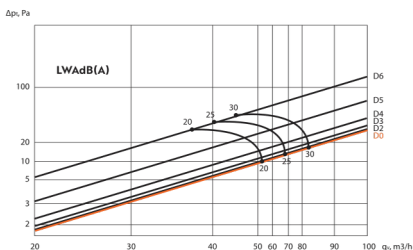
LINEO 600, 20 mm plyšys (oro ištraukimas)
